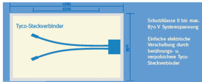
Maßzeichnung Tyco-Steckverbinder P210-60 GET AK
